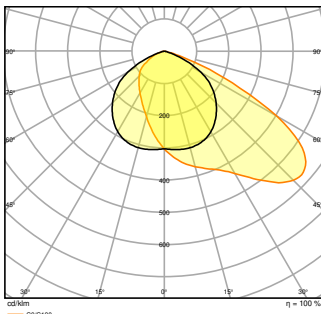
FL PFM 290W 3000K ASYM 55x110 BK
